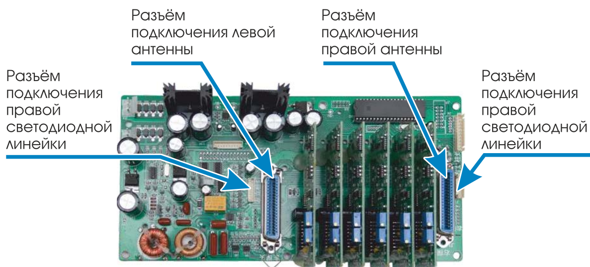
Рисунок 4. Материнская плата.
